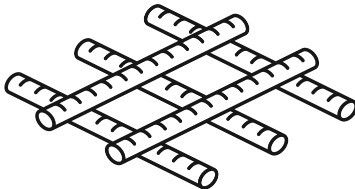
TIED CAGE
